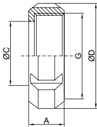
圆螺母长型 Round Nut(Long-type)
